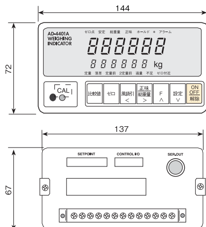
外形寸法図 ※詳しくは、AD-4401Aの取扱説明書もしくは簡易取扱説明書をご参照ください。
