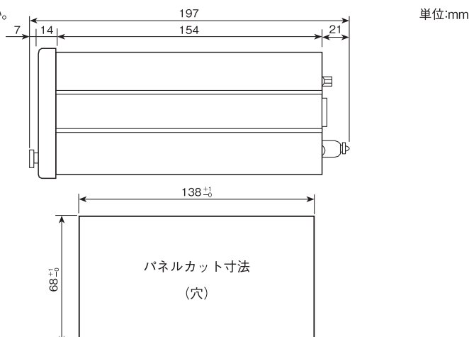
外形寸法図 ※詳しくは、AD-4401Aの取扱説明書もしくは簡易取扱説明書をご参照ください。
