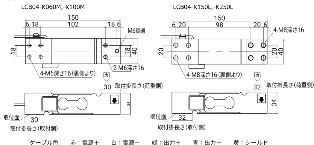
外形寸法図
