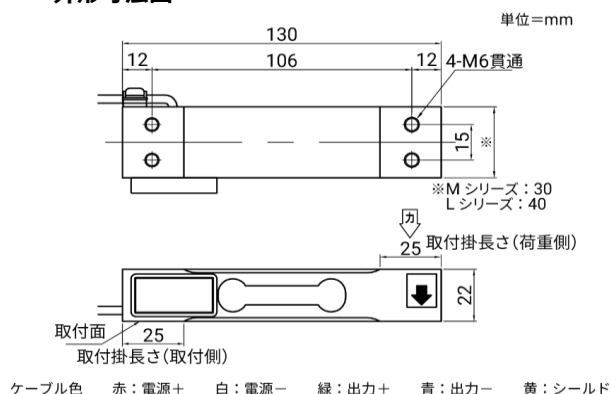
外形寸法図
