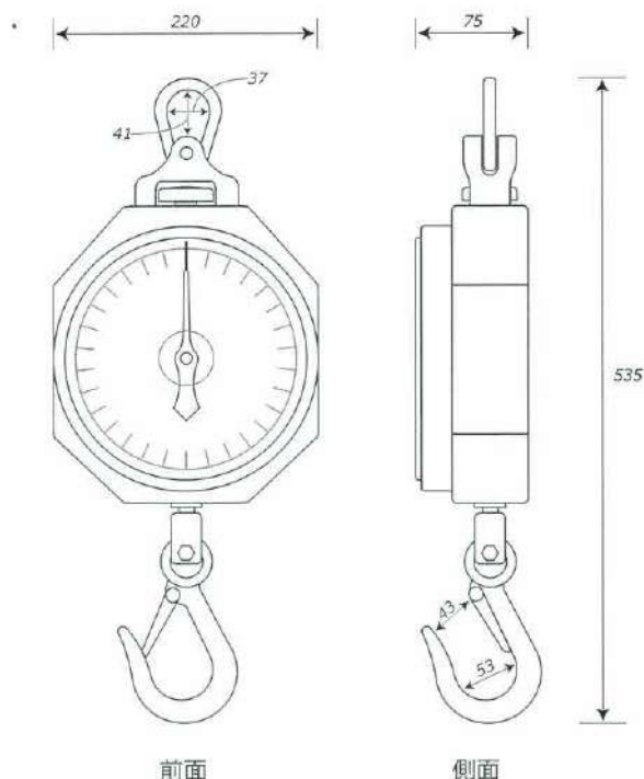
RTU 200kg/250kg/300kg 外形寸法図 単位 mm
