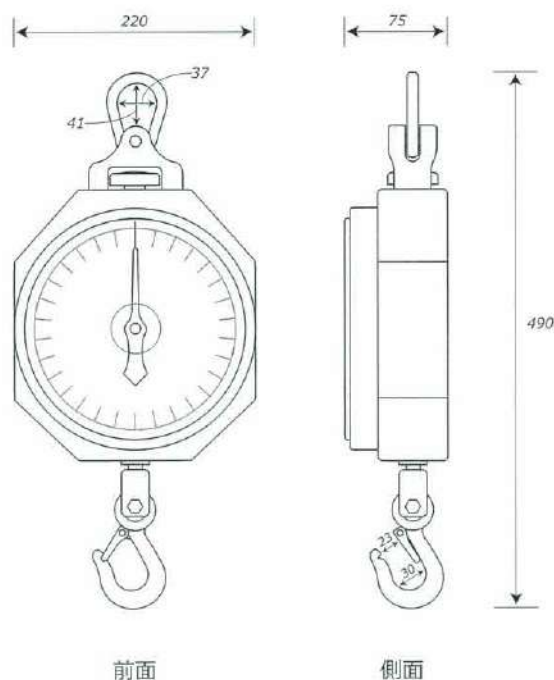
RTU 30kg/60kg/120kg 外形寸法図 単位 mm
